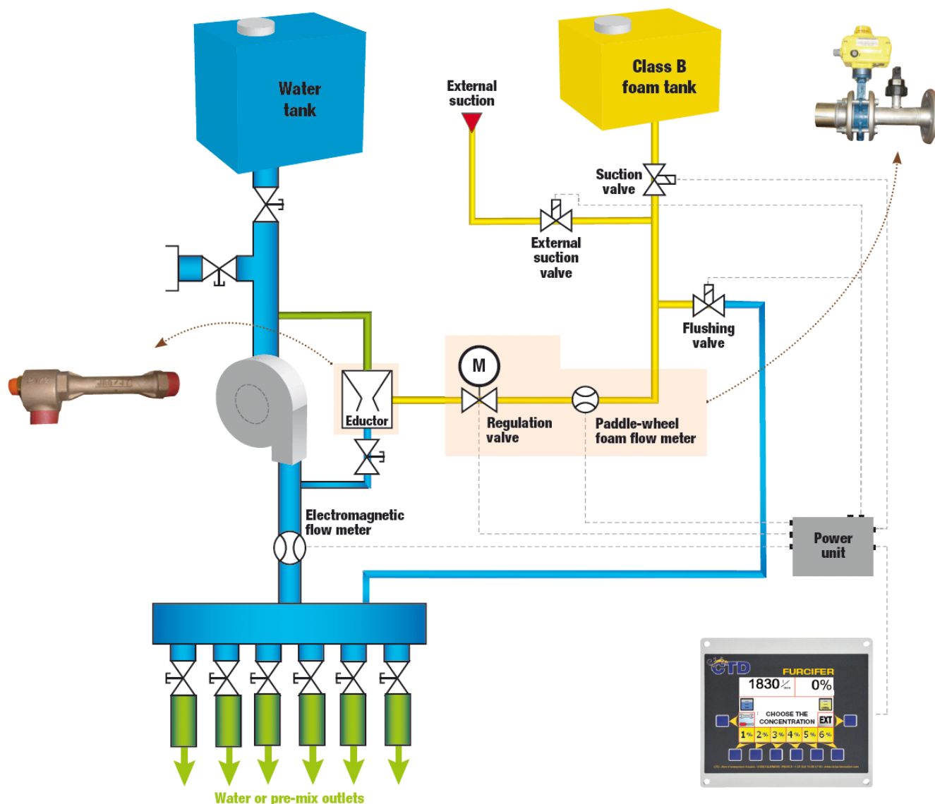
سیستم دیجیتال Hydromante جهت تصحیح تناسب‌سازهای پمپ فوم با بالانسر
